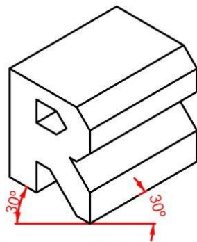
Isométrica
